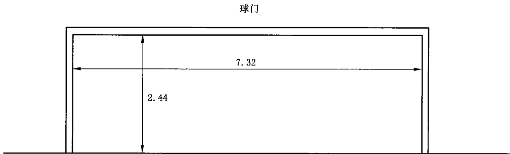
图 2 11人制足球场球门正面图
