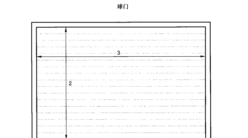
图 5 5 人制足球场地球门正面图
