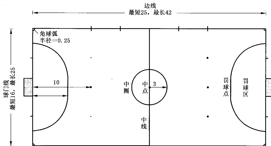
图 3 5人制足球场平面图
